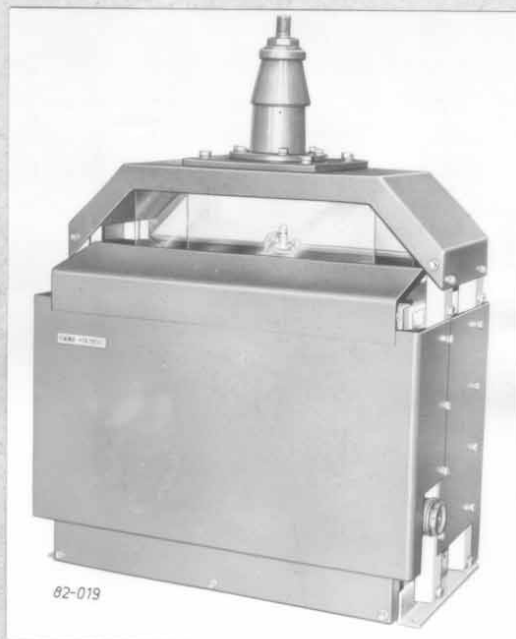
KTA 1300 Antennenhalterung mit Isolator der 6 m-Stabantenne
